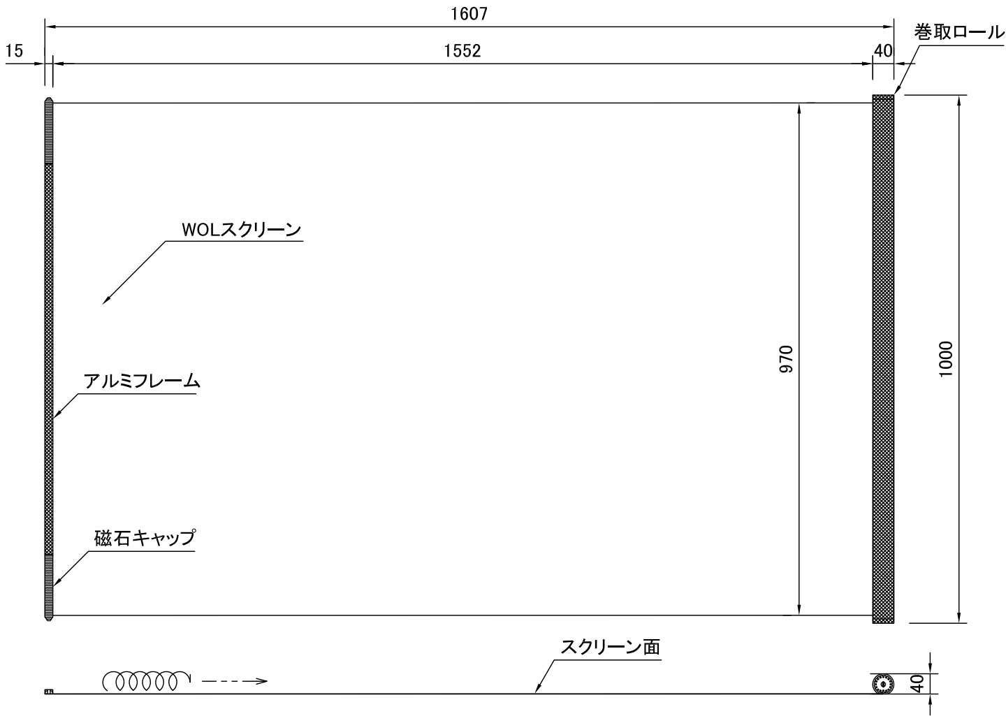
マグネットスクリーン S=1/10
