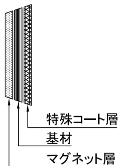
WOLスクリーン構造図
