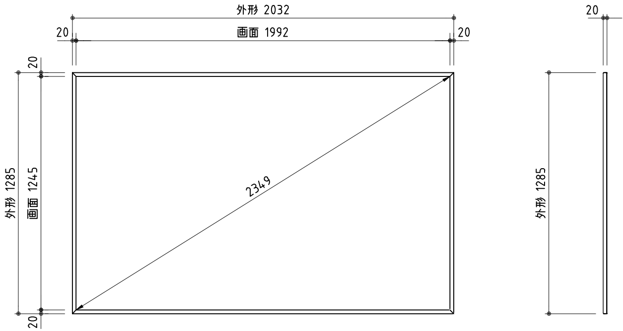
外観図(正面) S=1/20
