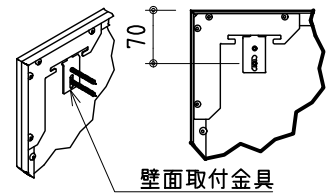
A部 詳細(1:10)
