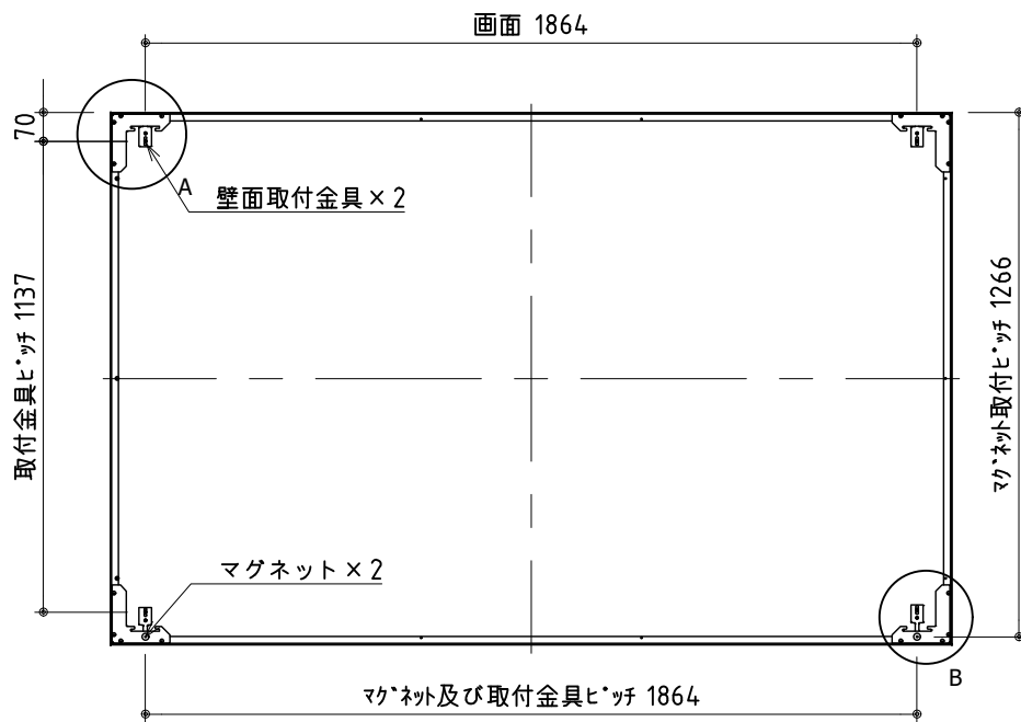
外観図(背面) S=1/20
