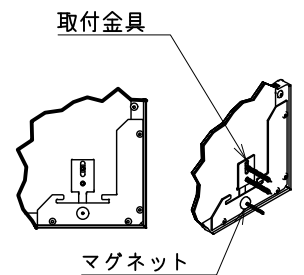
B部 詳細(1:10)
