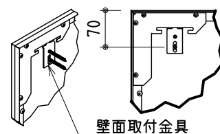
A部 詳細(1:10)
