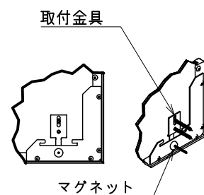
B部 詳細(1:10)
