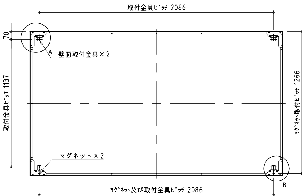
外観図(背面) S=1/20
