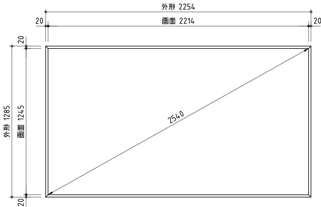
外観図(正面) S=1/20
