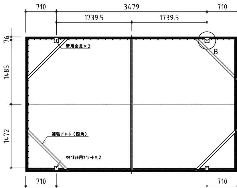
外観図(背面) S=1/50
