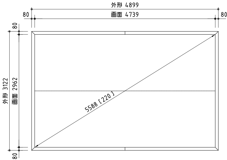
外観図 S=1/50
