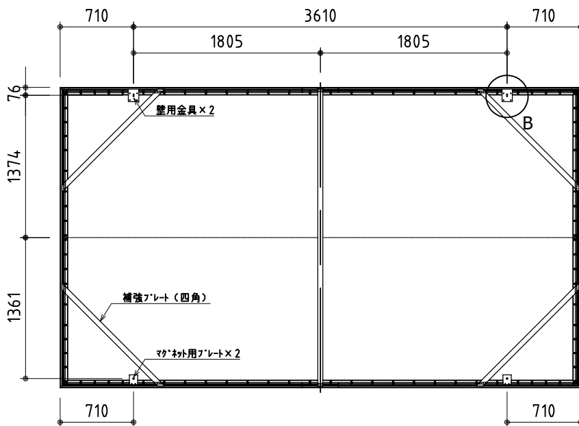
外観図(背面) S=1/50
