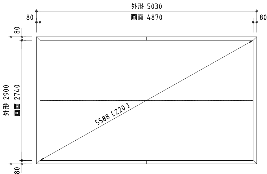
外観図 S=1/50
