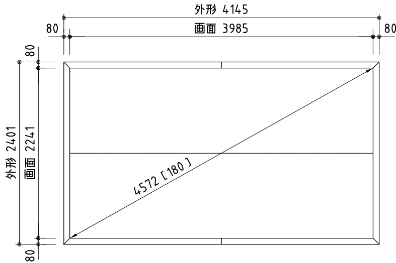
外観図 S=1/50
