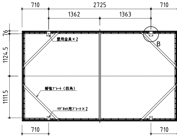
外観図(背面) S=1/50
