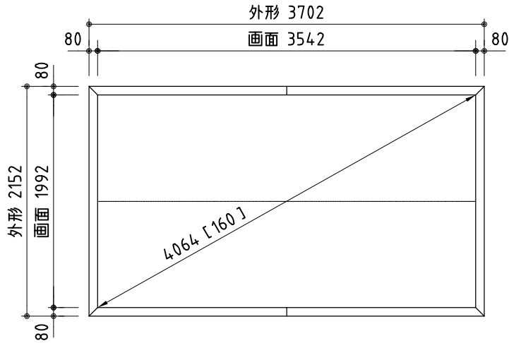
外観図 S=1/50
