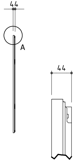
A部 詳細(1:5)
