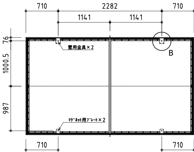
外観図(背面) S=1/50
