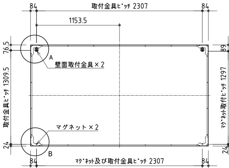
外観図(背面) S=1/30
