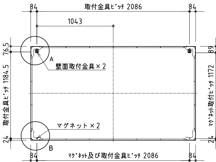
外観図(背面) S=1/30
