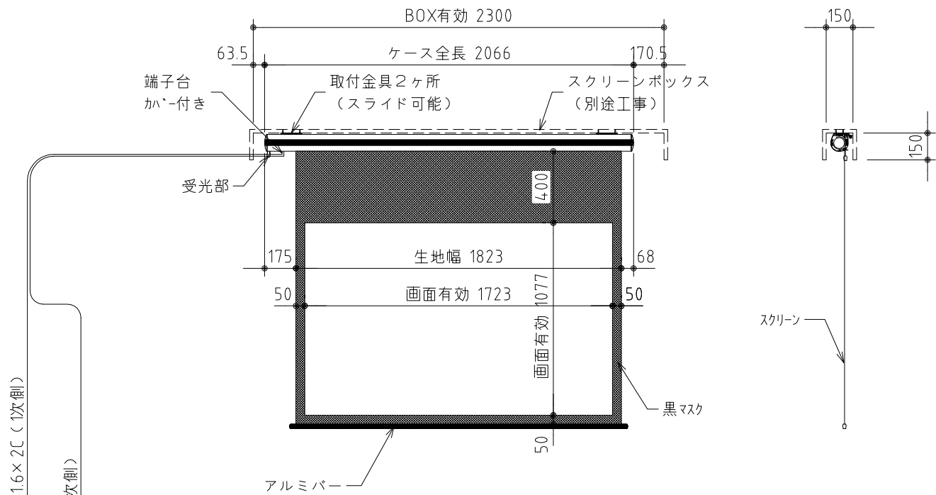
外観図 1/30
