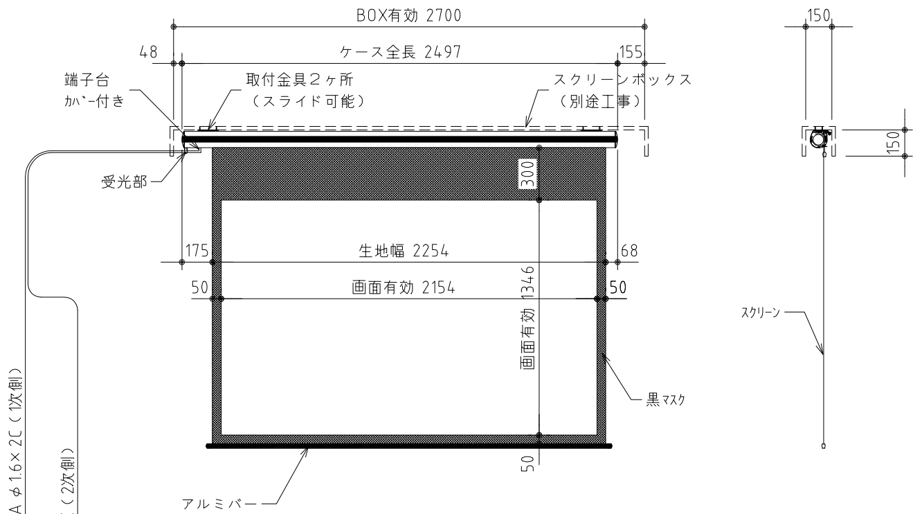
外観図 1/30
