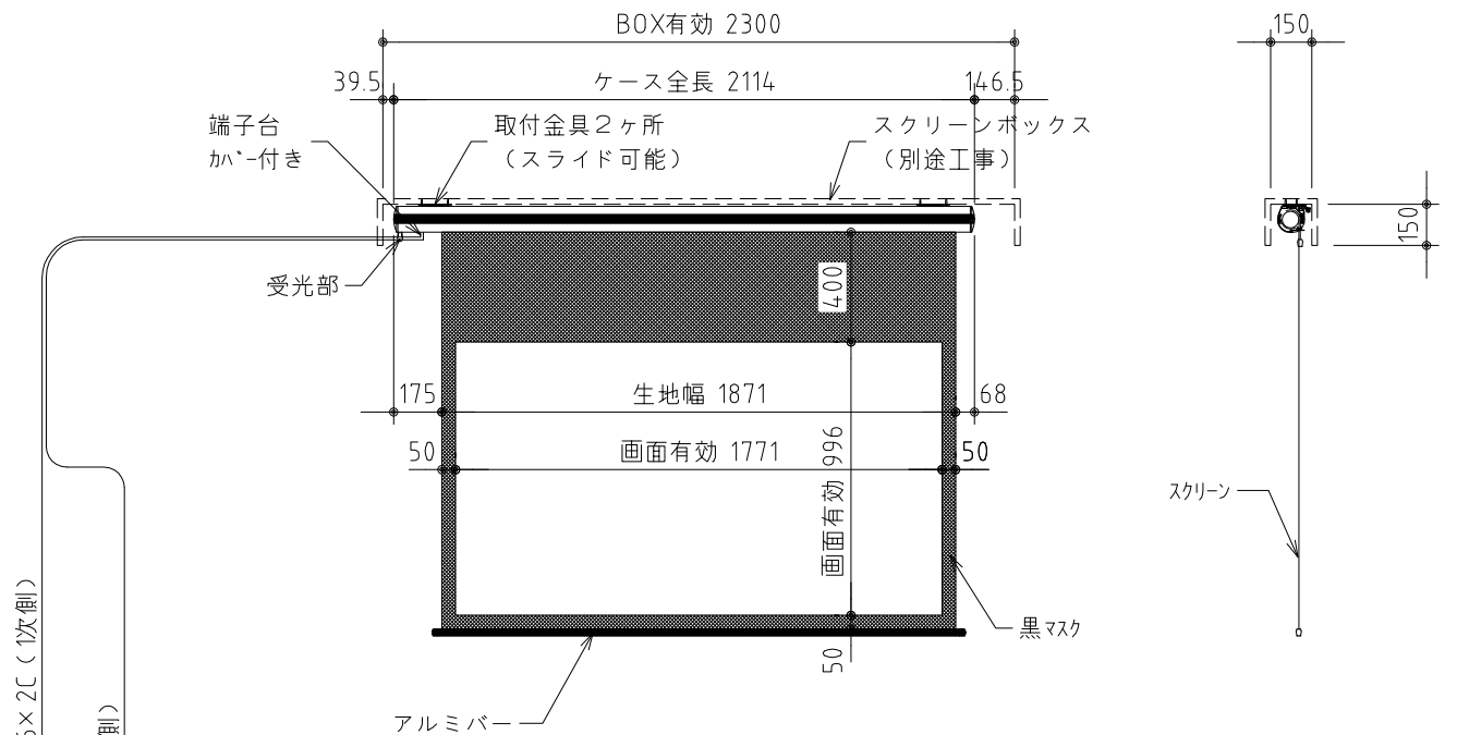
外観図 1/30
