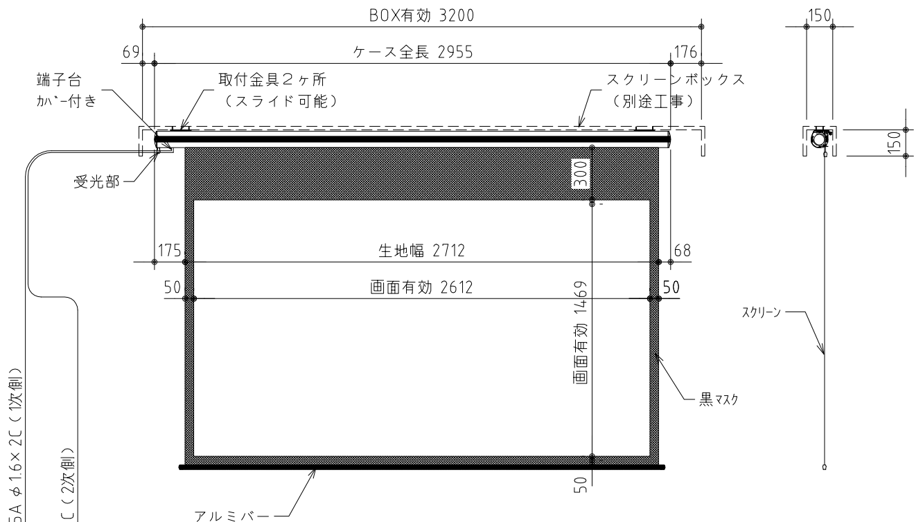
外観図 1/30
