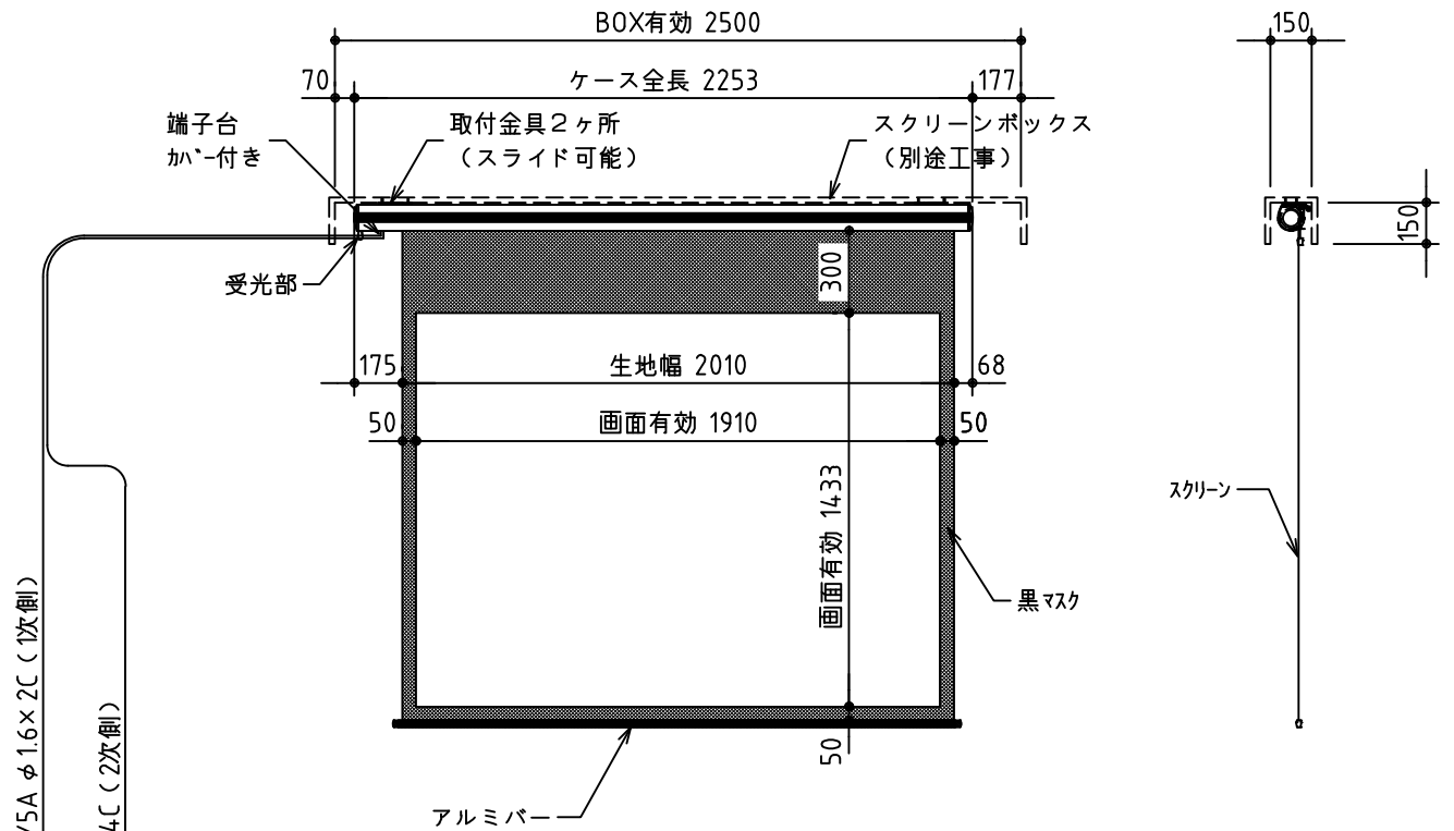
外観図 1/30
