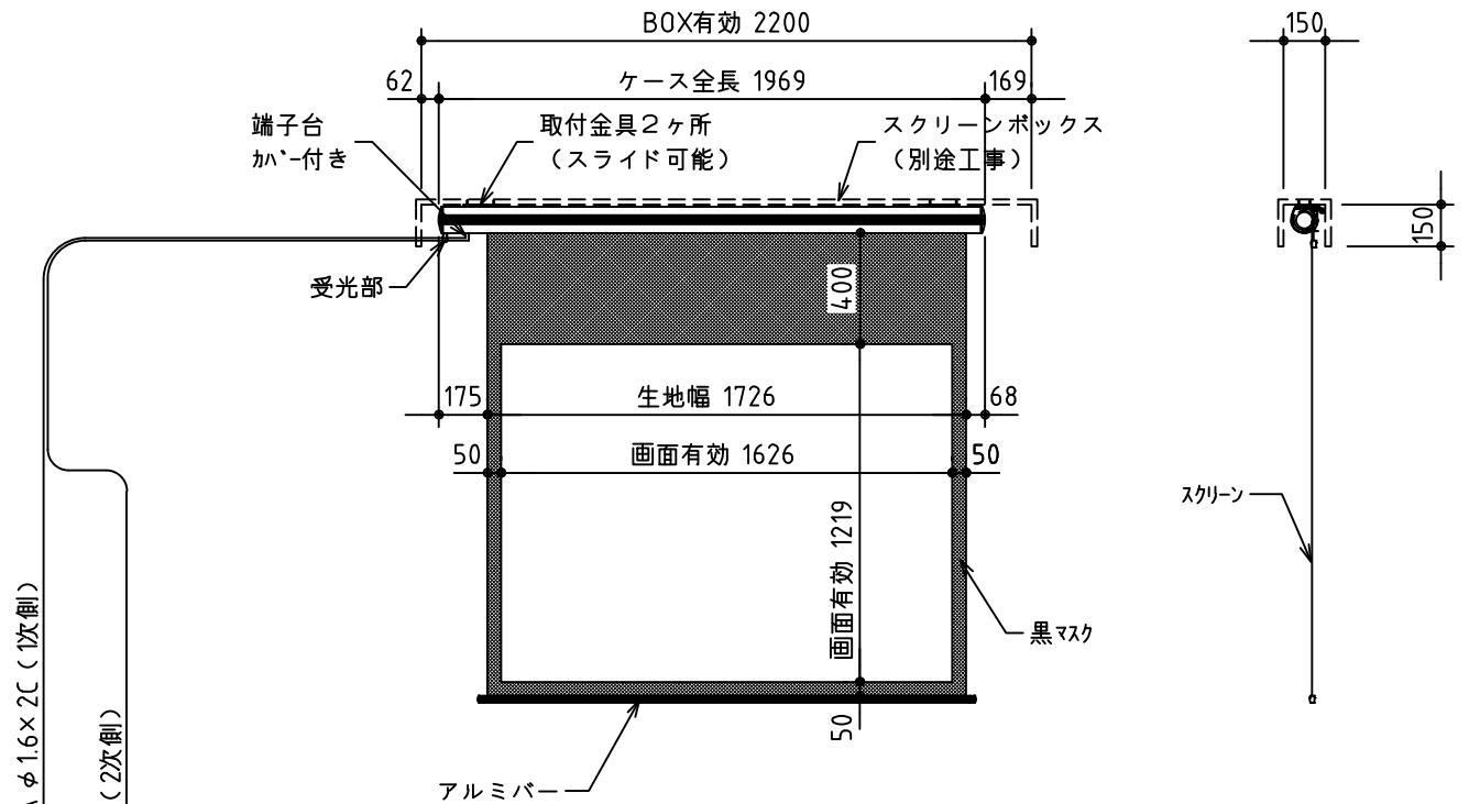
外観図 1/30
