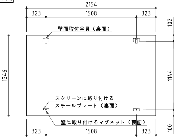
壁面取付金具詳細 (1/5)
