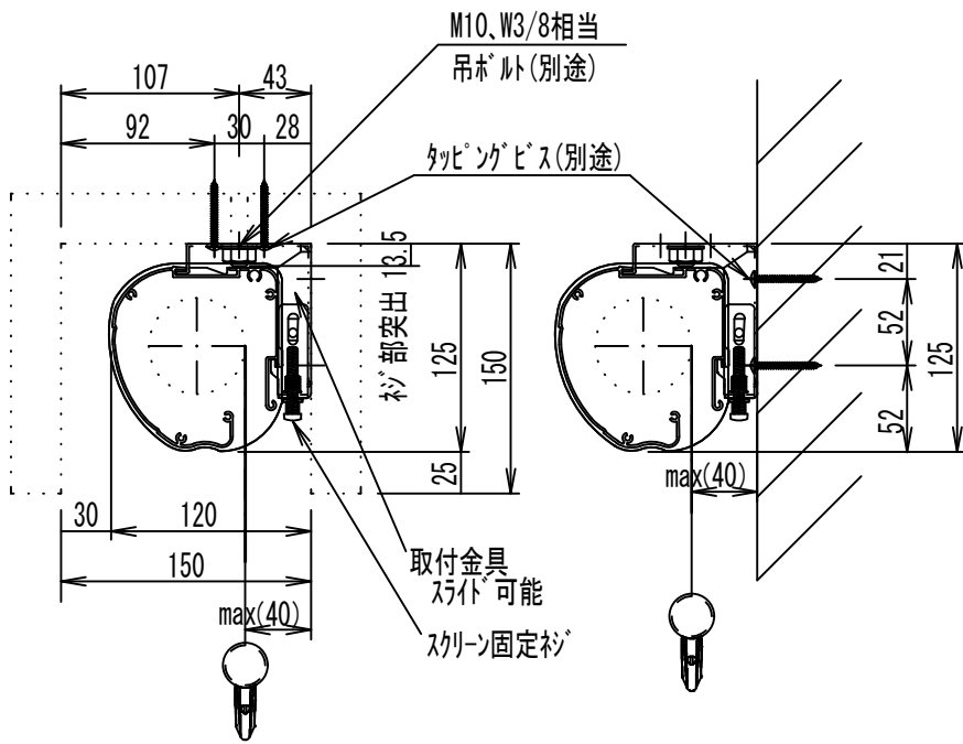
ボックス取付時 S=1/5
