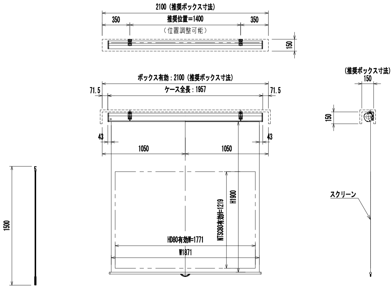
外観図 S=1/30
