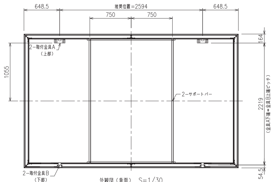
外観図（背面） S=1/30
