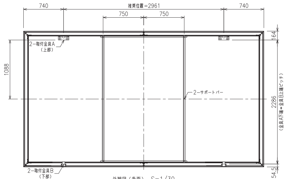
外観図（背面） S=1/30
