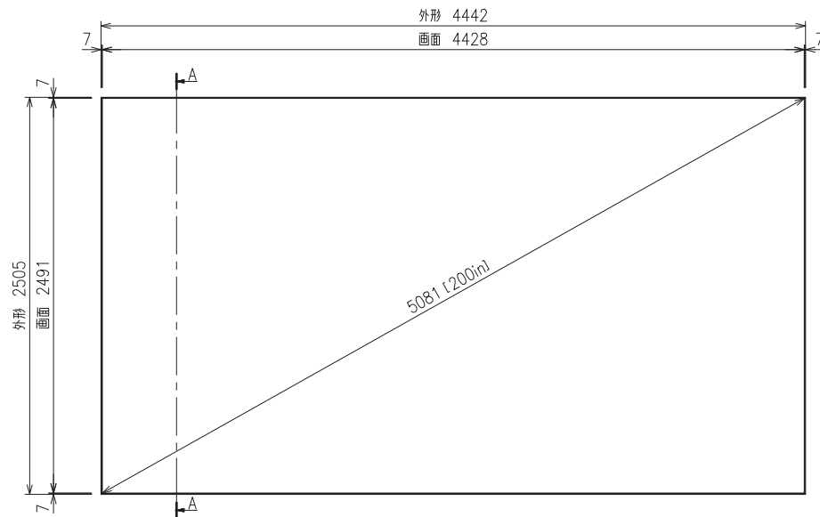
外観図（正面） S=1/30
