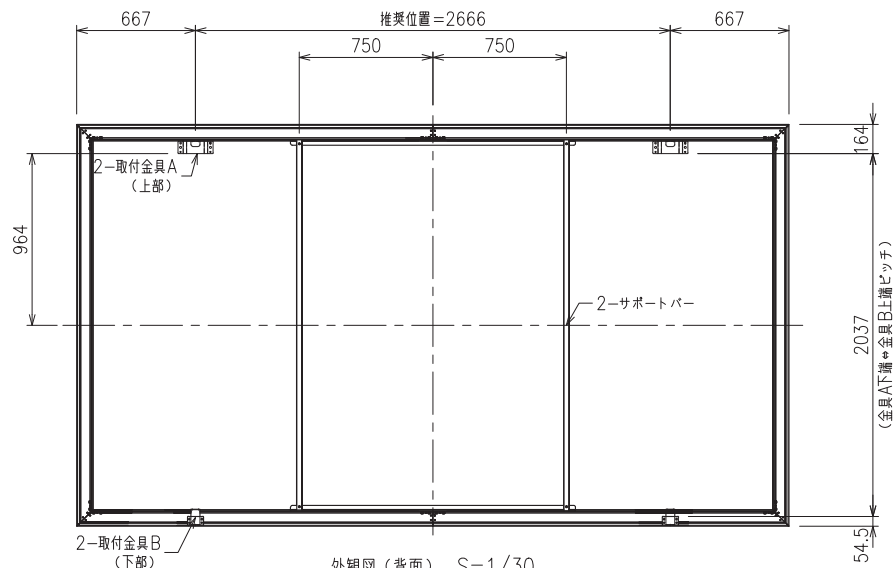
外観図（背面） S=1/30
