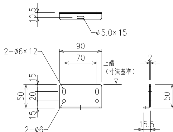
壁取付金具B 詳細 S= 1/5
