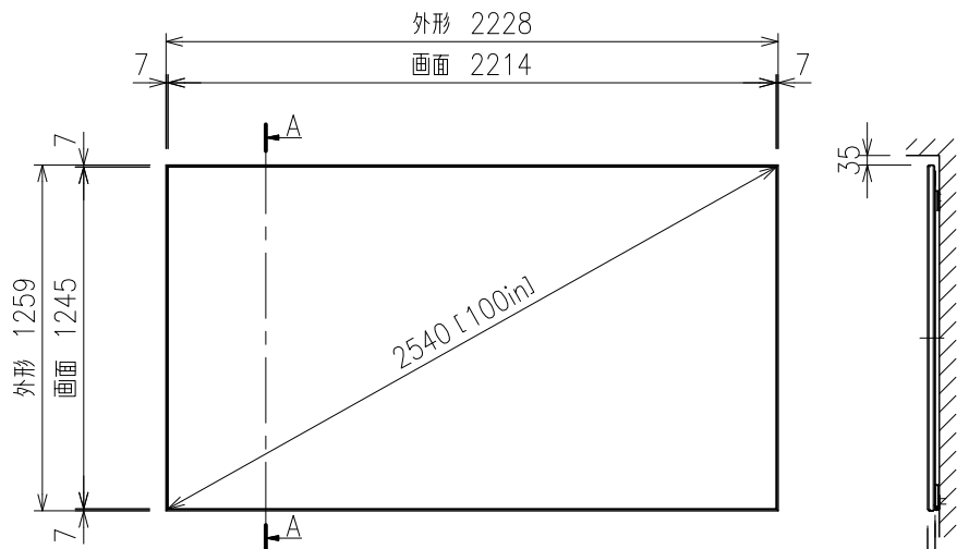
外観図（正面） S=1/30
