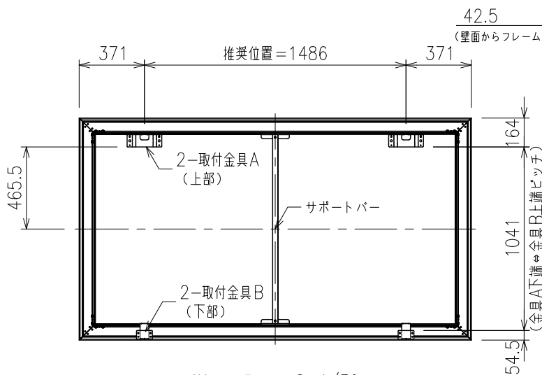
外観図（背面） S=1/30
