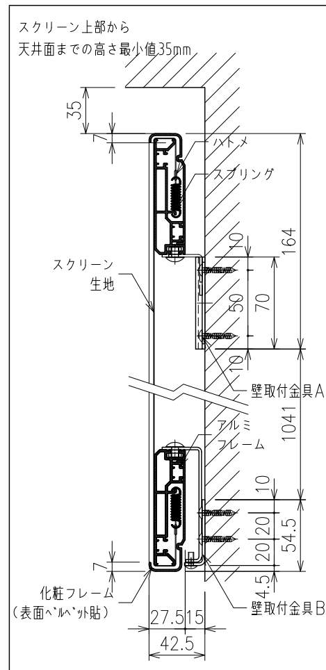
A断面詳細 S=1/4
