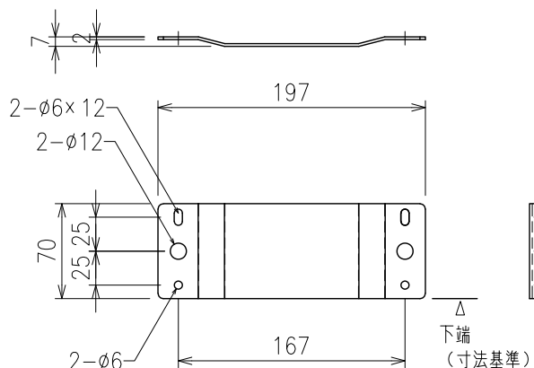
壁取付金具A 詳細 S= 1/5
