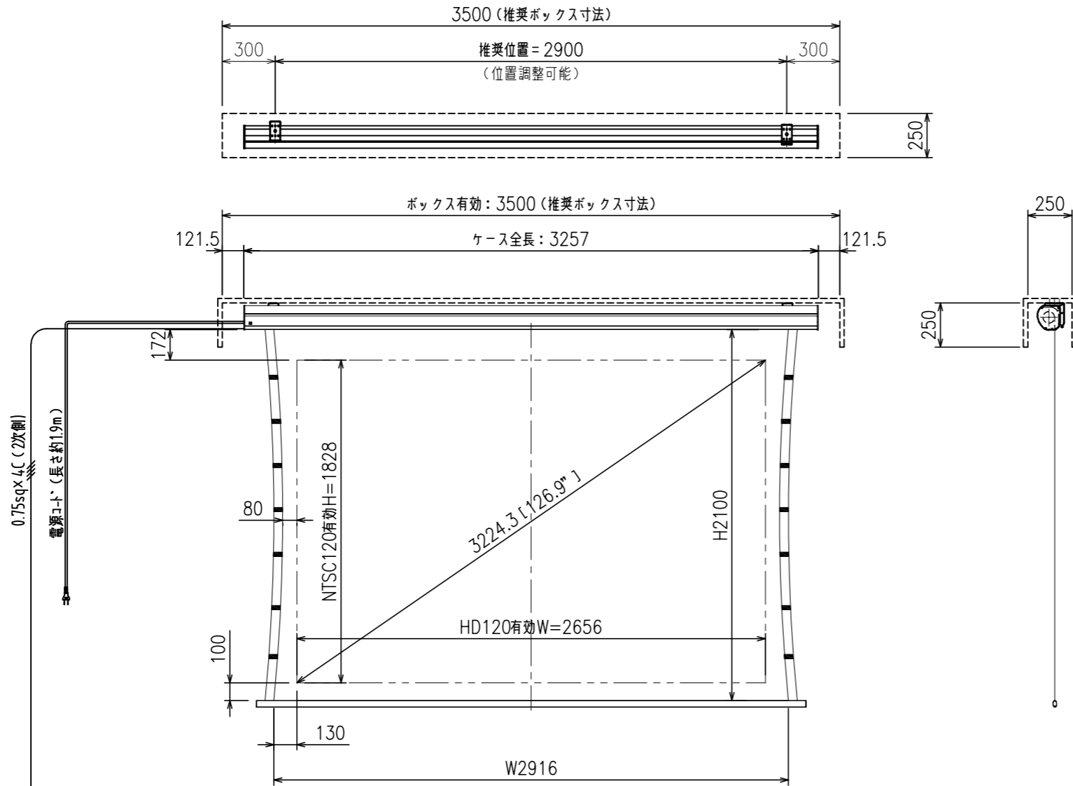
外觀図 S=1/30
