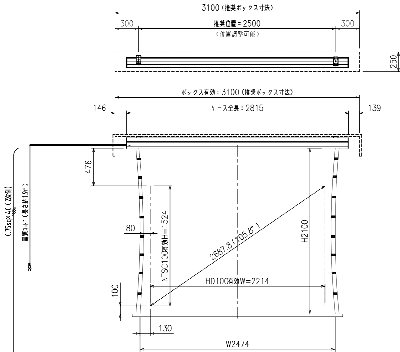
外觀図 S=1/30
