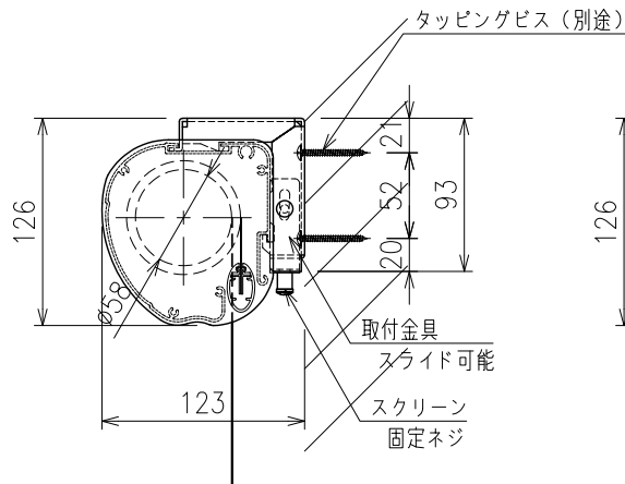
壁面取付時 S=1/5
