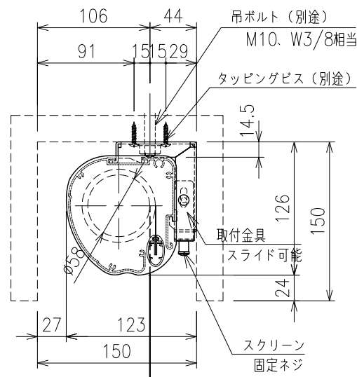
ボックス取付時 S=1/5
