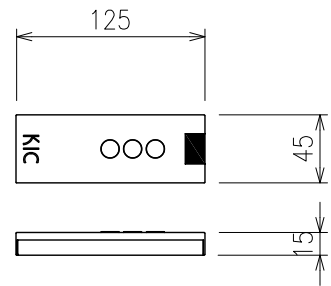
赤外線ワイヤレスリモコン S=1/5
