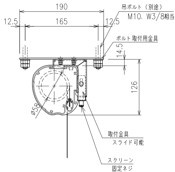
ボックス取付時 S=1/5
