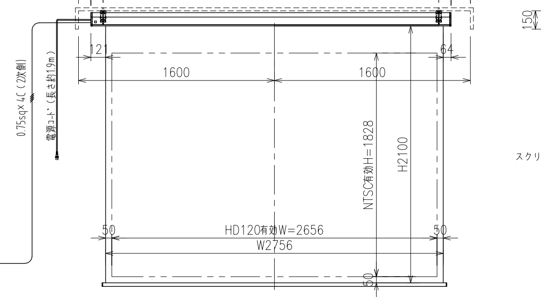
外観図 S=1/30
