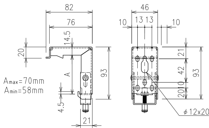
取付金具 S=1/6
