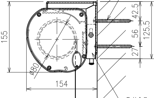
壁面取付時 S=1/5
