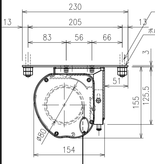
ボルト吊り取付時 S=1/5
