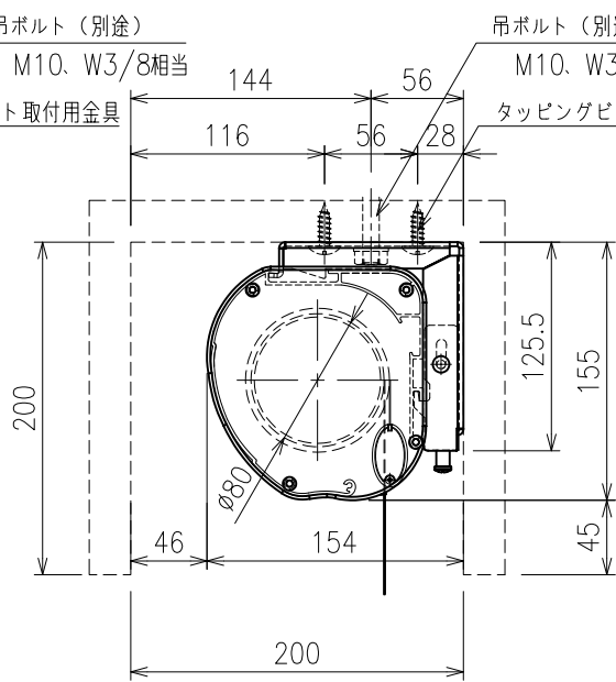
ボックス取付時 S=1/5
