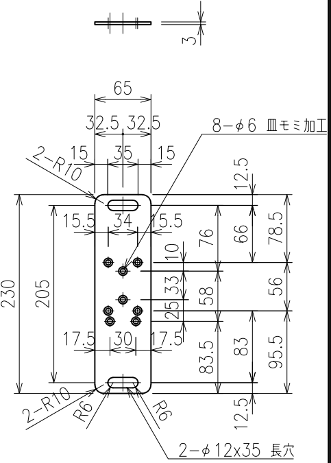
<ボルト取付用金具>
