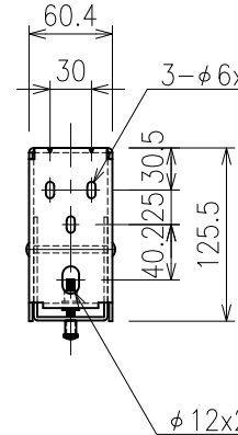
取付金具 S=1/6
