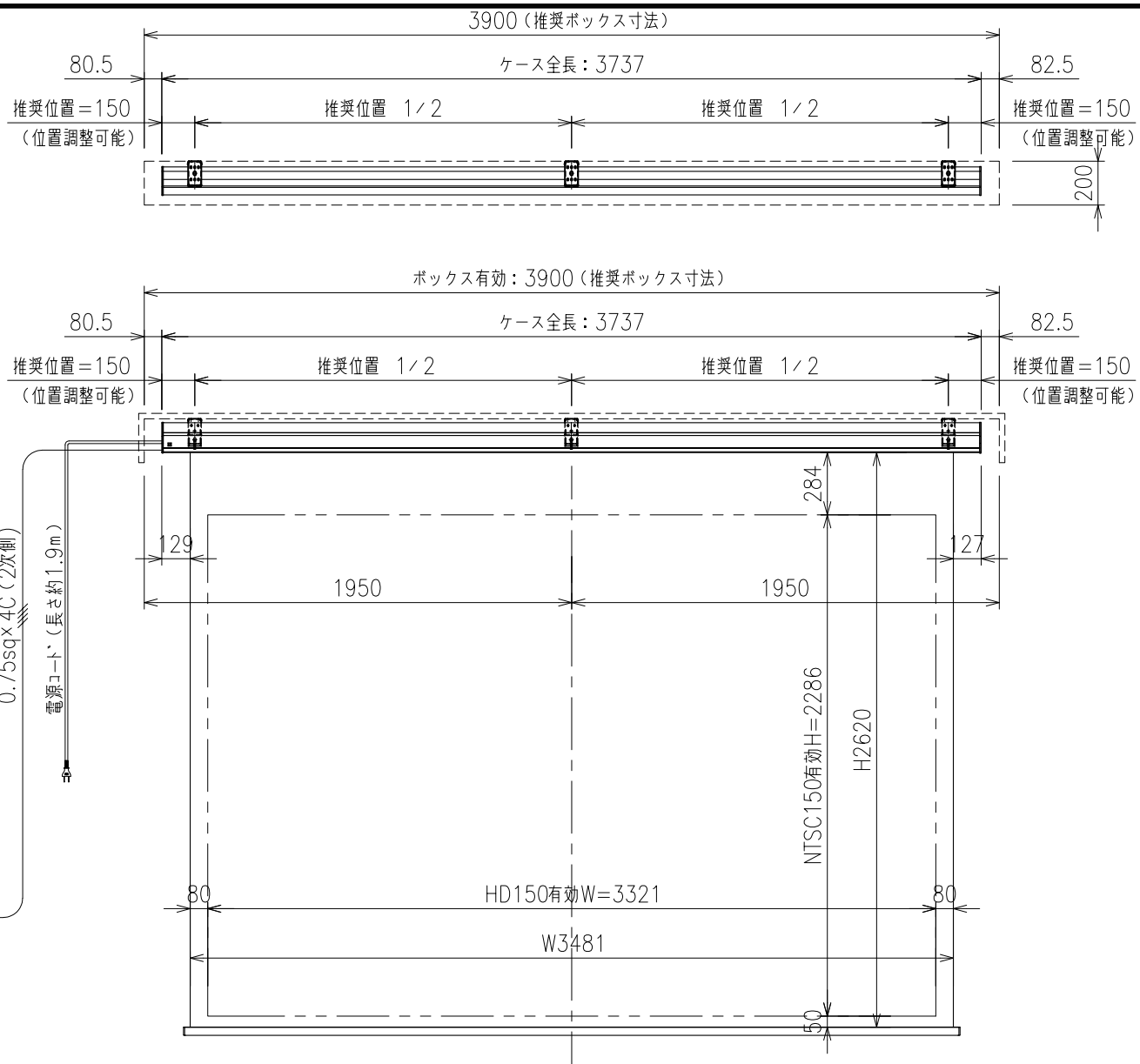
外観図 S=1/30
