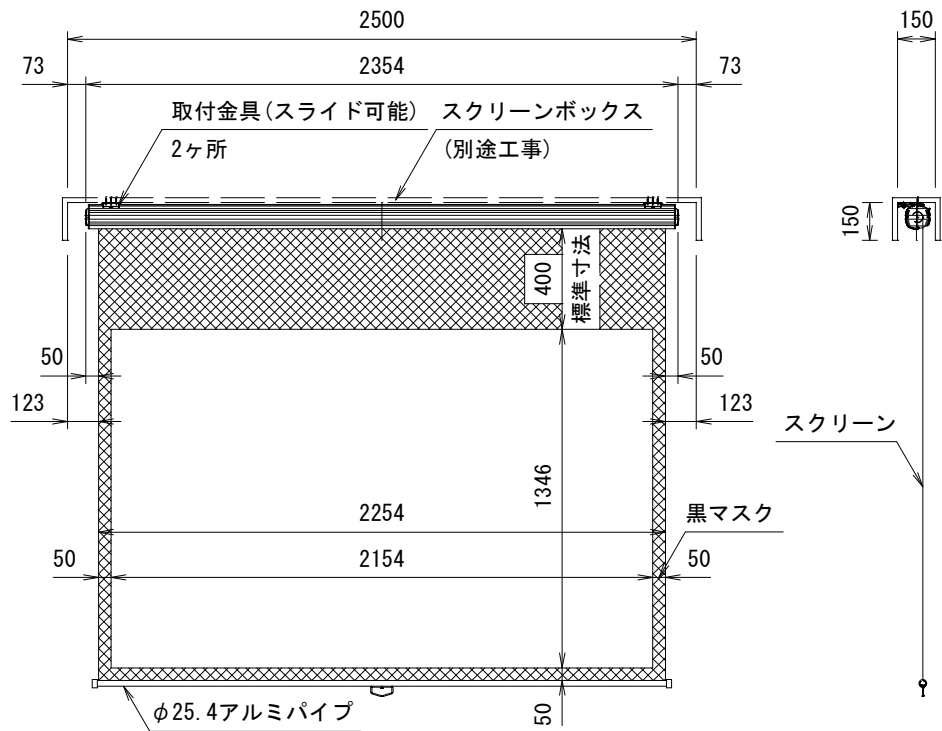
外観図 S=1/30
