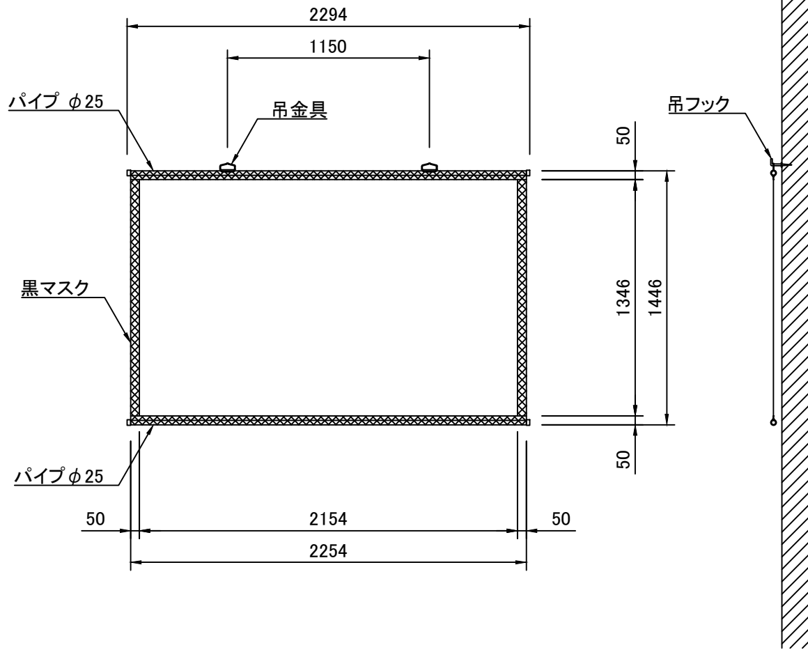
外観図 S=1/30
