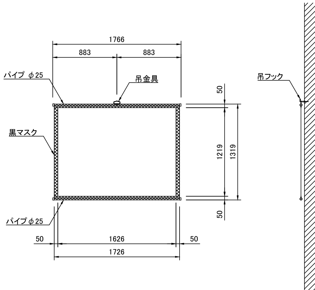
外観図 S=1/30
