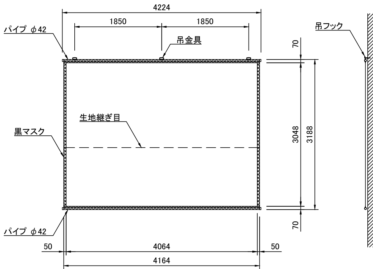
外観図 S=1/50
