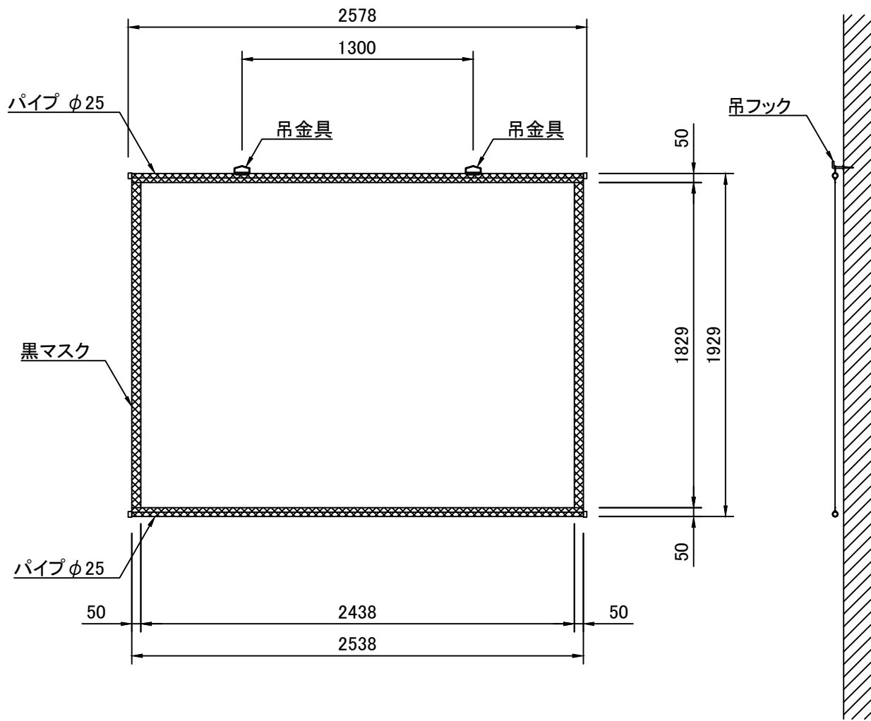
外観図 S=1/30
