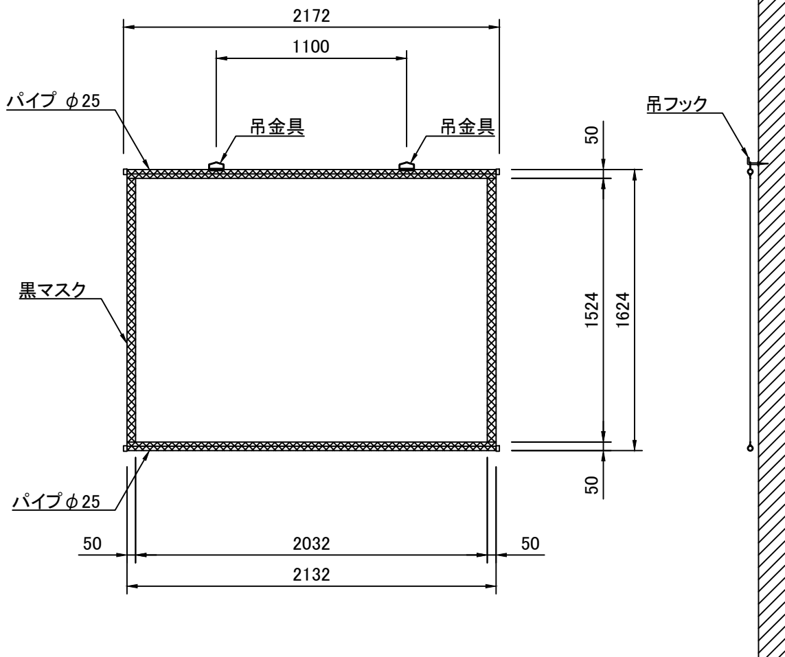
外観図 S=1/30
