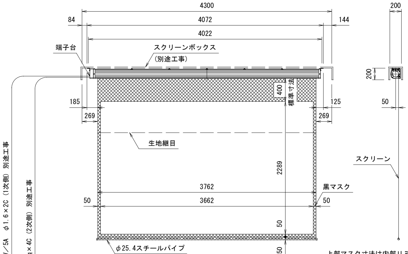
外觀図 S=1/40
