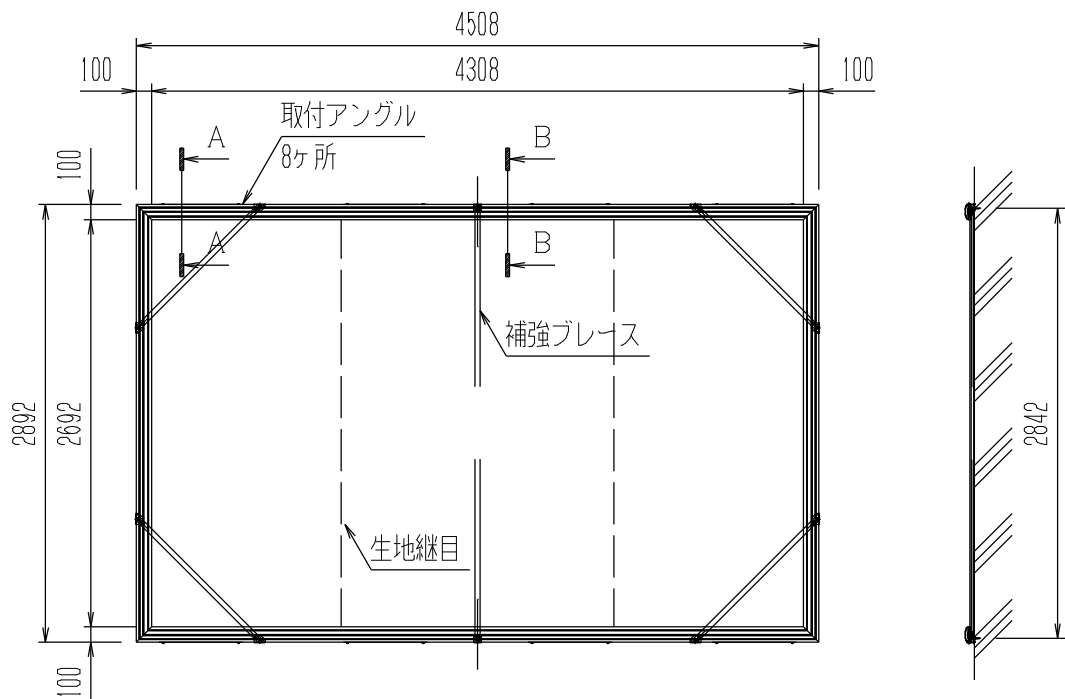
外觀図 S=1/50
