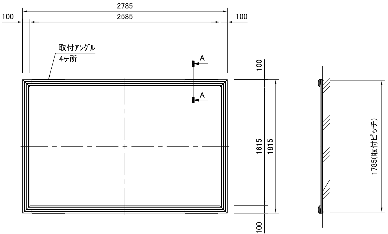
外観図 S=1/30
