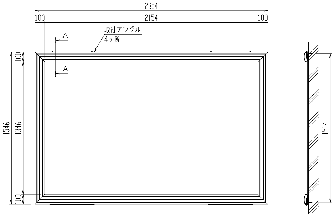
外觀図 S=1/20
