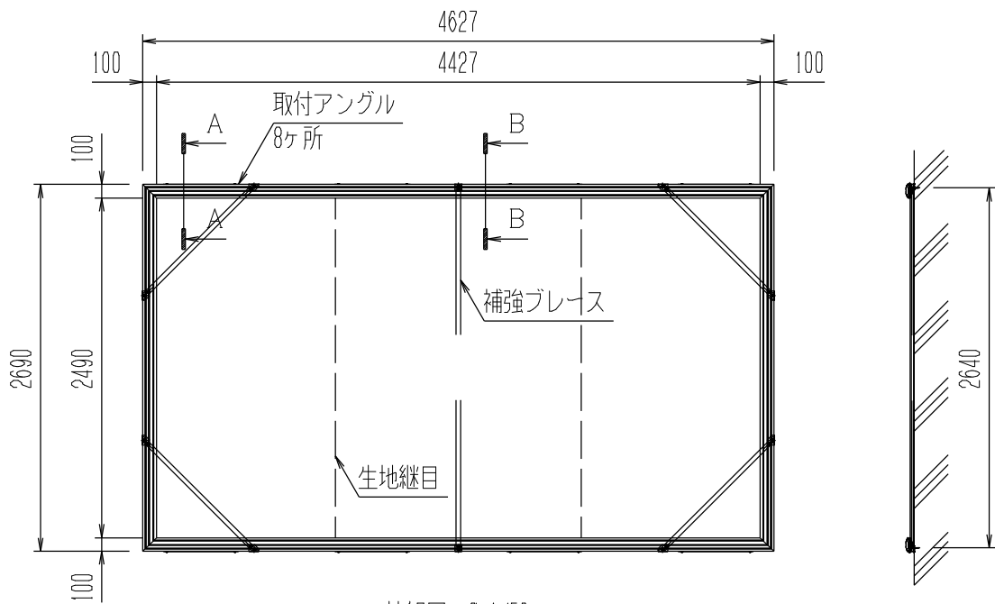
外観図 S=1/50
