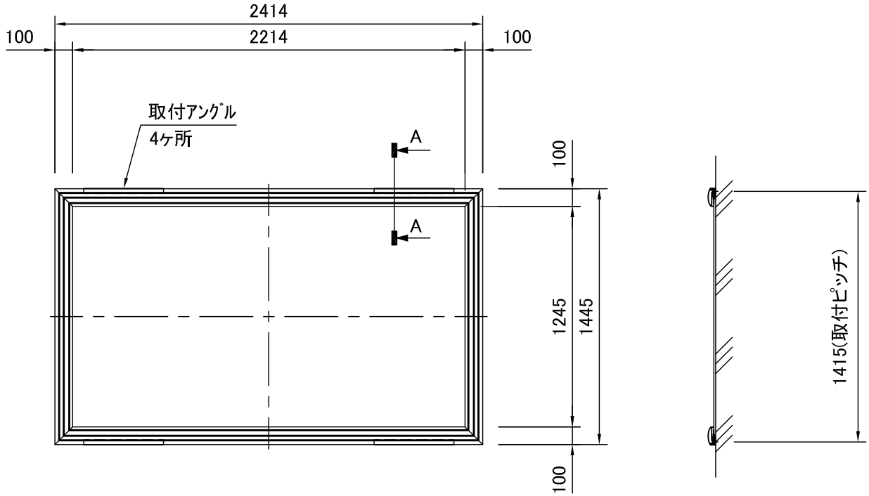
外観図 S=1/30
