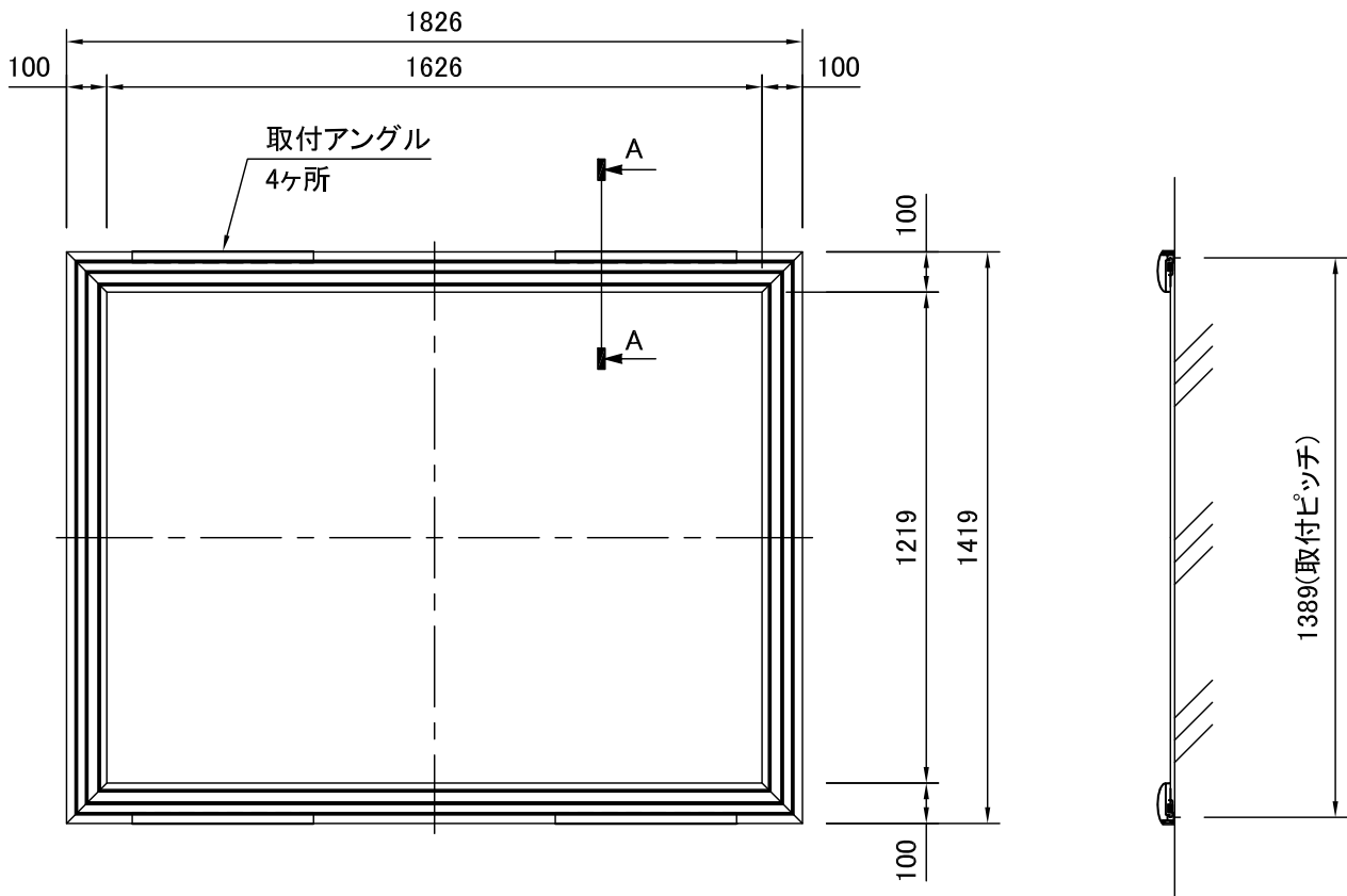
外観図 S=1/20
