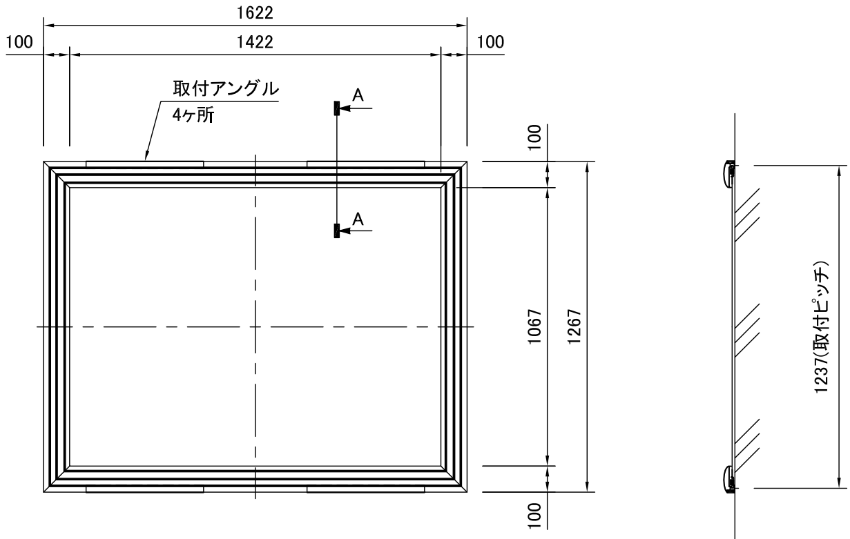
外觀図 S=1/20
