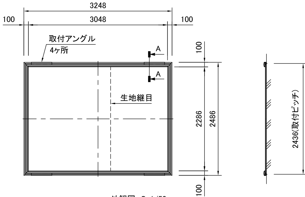
外観図 S=1/50
