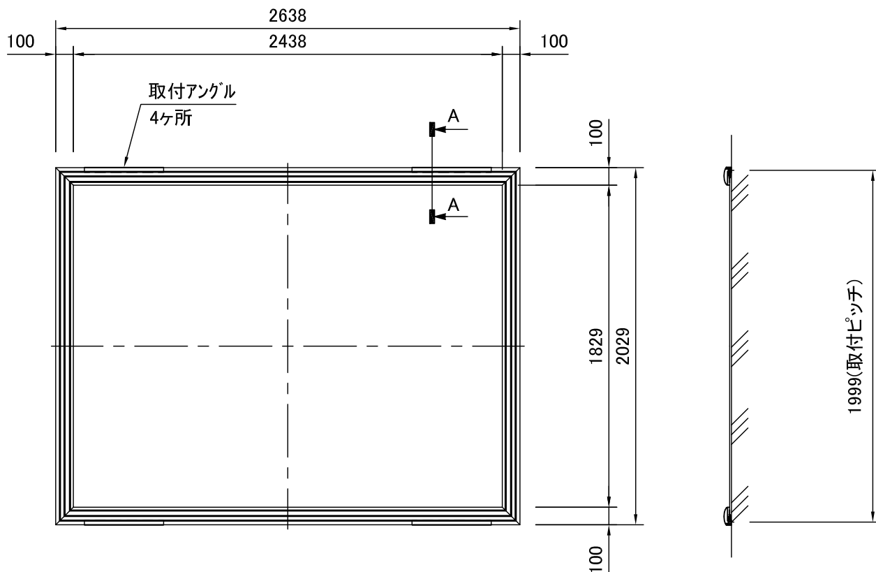
外観図 S=1/30
