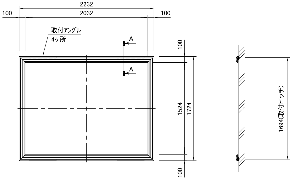
外観図 S=1/30
