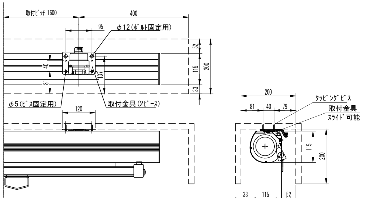
詳細図 1/8
