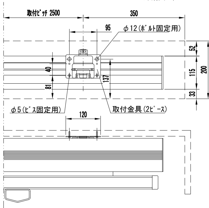
外観図 1/30
