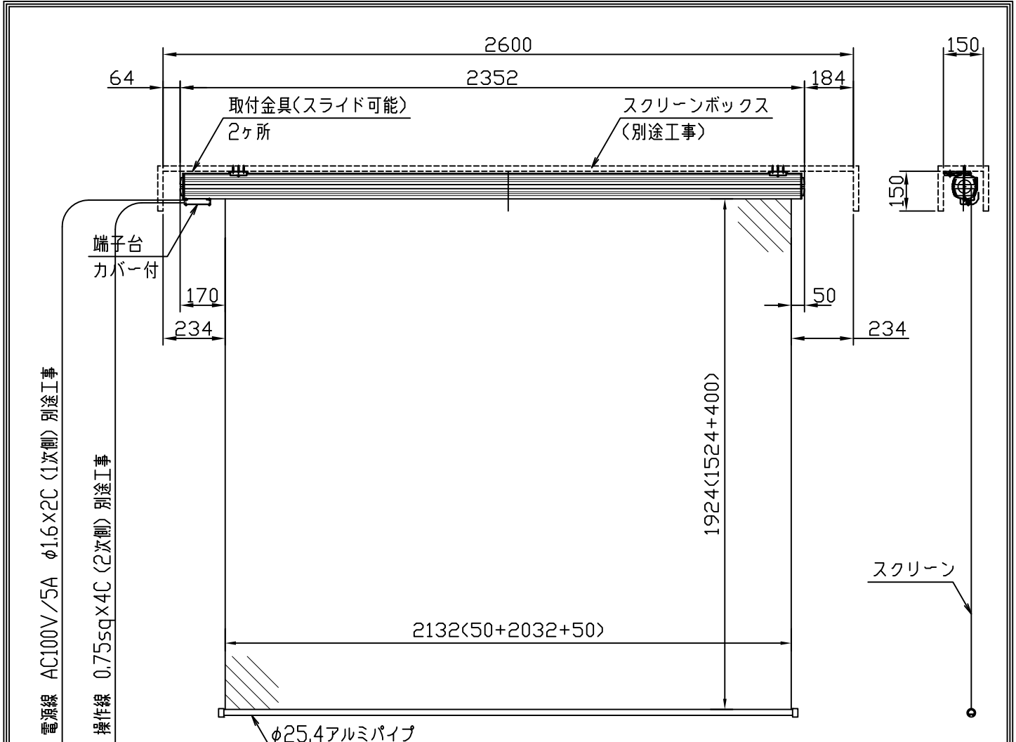
外觀図 S=1/20
