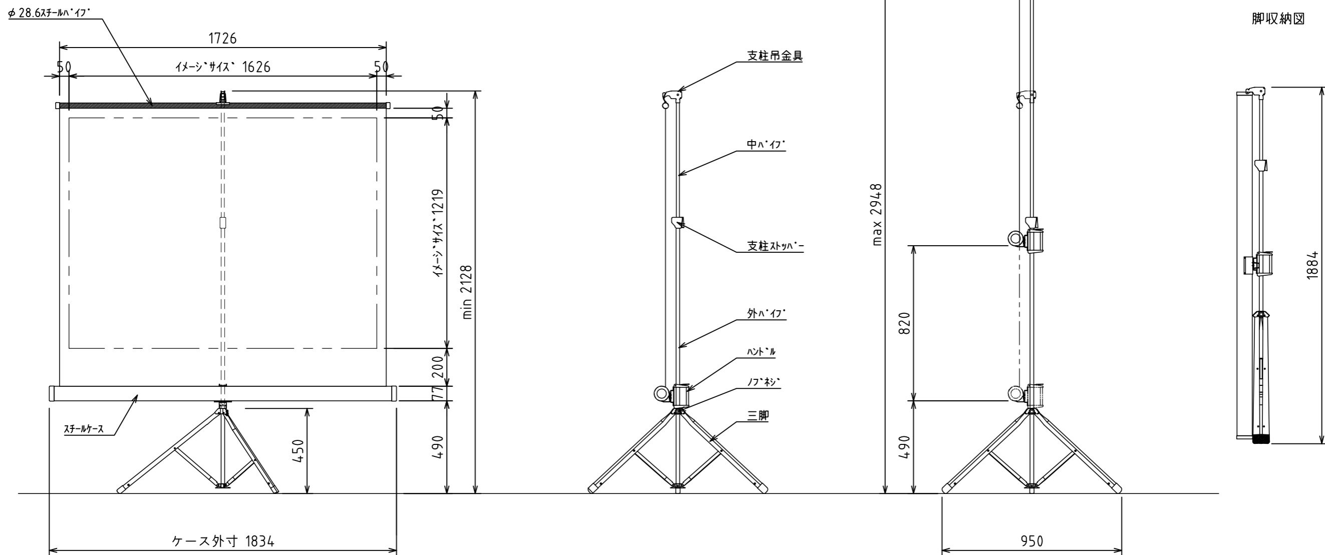
外観図 1/20
