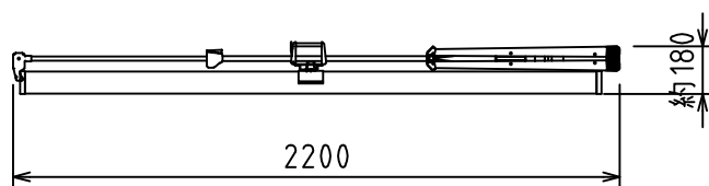
脚収納図
