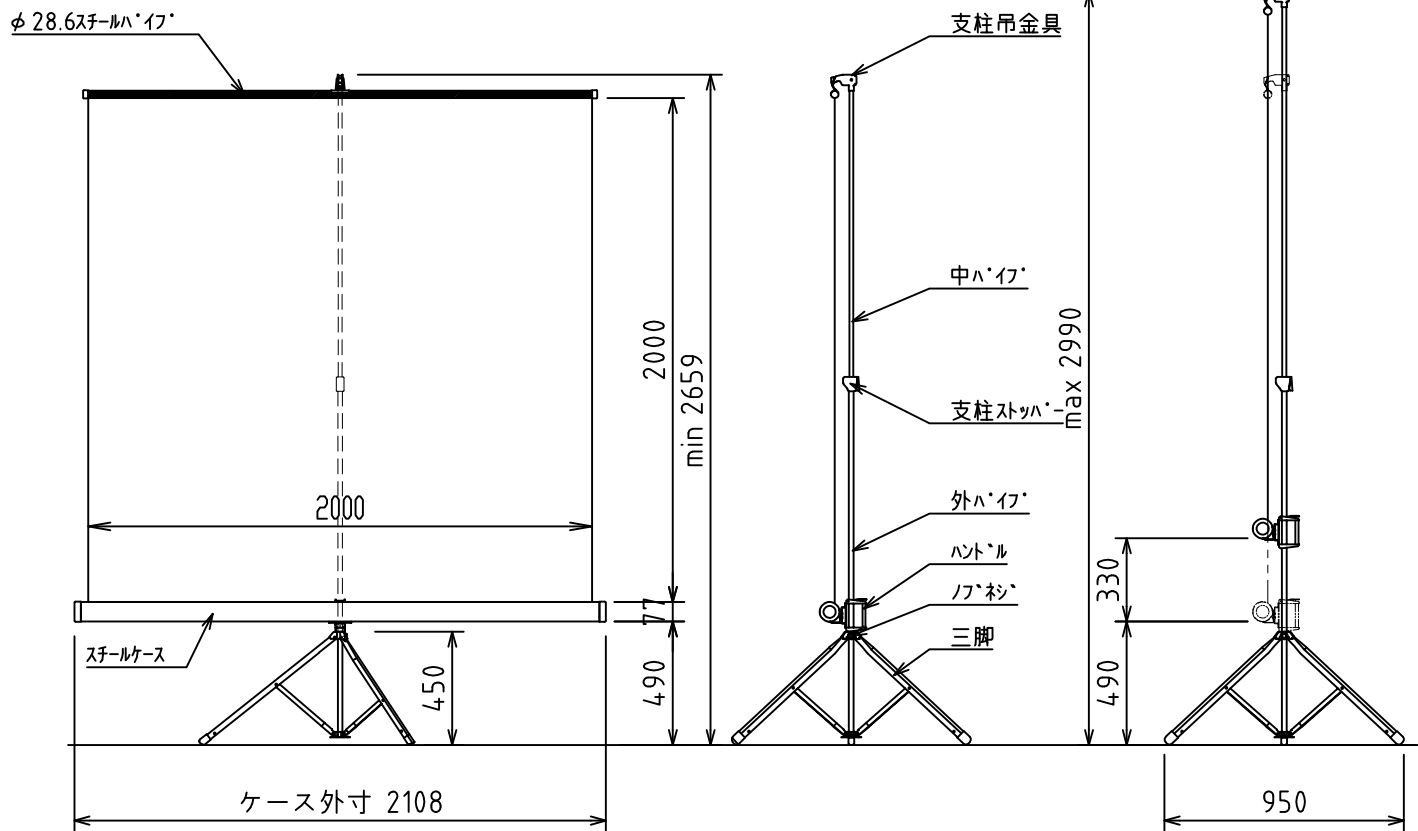
外観図 1/30
