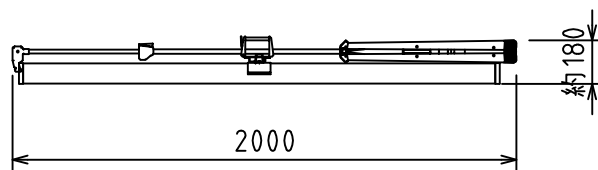
脚収納図
