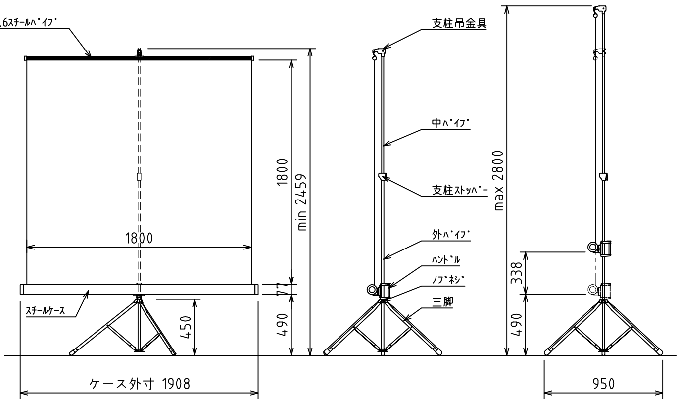
外観図 1/30
